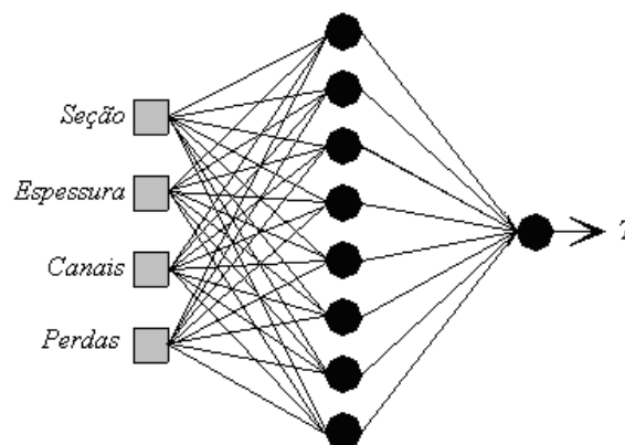
Figura 3.7 - Arquitetura da rede Perceptron.
