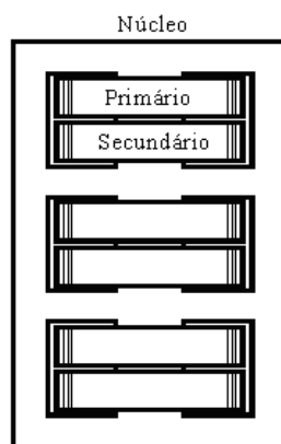
Figura 2.2 - Transformador trifásico do tipo de núcleo envolvente.
