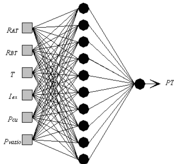
Figura 3.11 - Arquitetura da rede Perceptron para perdas totais.
