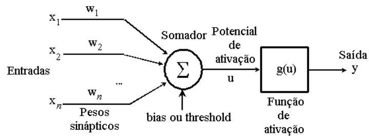
Figura 3.1 – Modelo geral do neurônio artificial.
