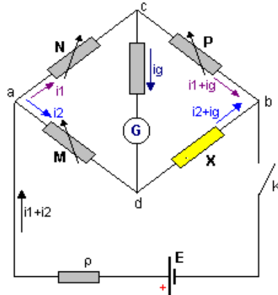
Figura 3.10 - Ponte de Wheatstone.
