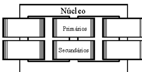
Figura 2.3 - Transformador trifásico do tipo de núcleo envolvido.
