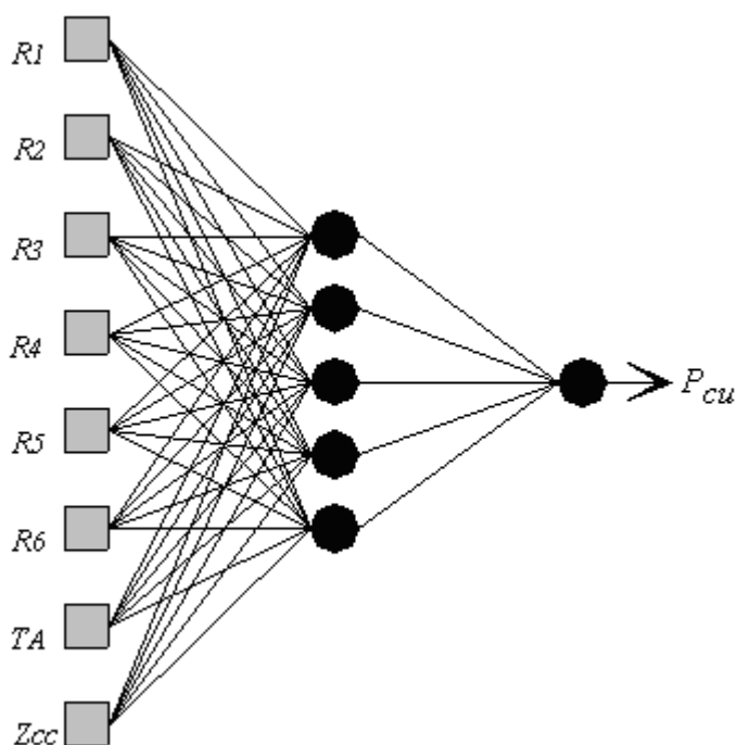
Figura 3.12 - Arquitetura da rede Perceptron para perdas no cobre.
