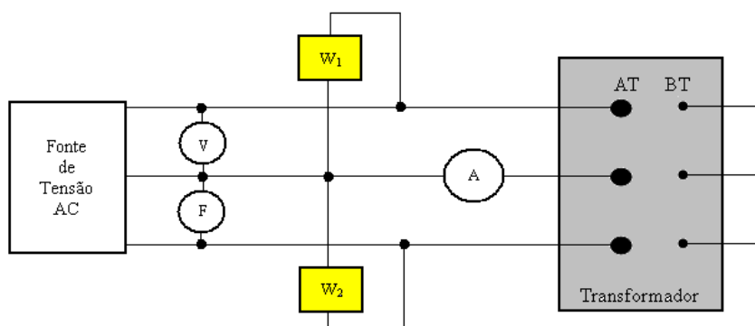
Figura 3.9 - Esquema do ensaio em curto circuito.
