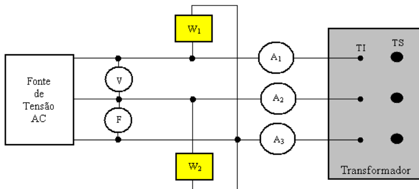
Figura 3.8 - Esquema do ensaio a vazio.
