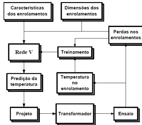
Figura 3.6 - Sistema proposto para a RNA.
