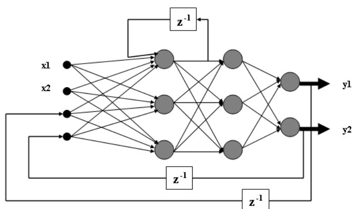
Figura 3.5 - Exemplo de rede recorrente.
