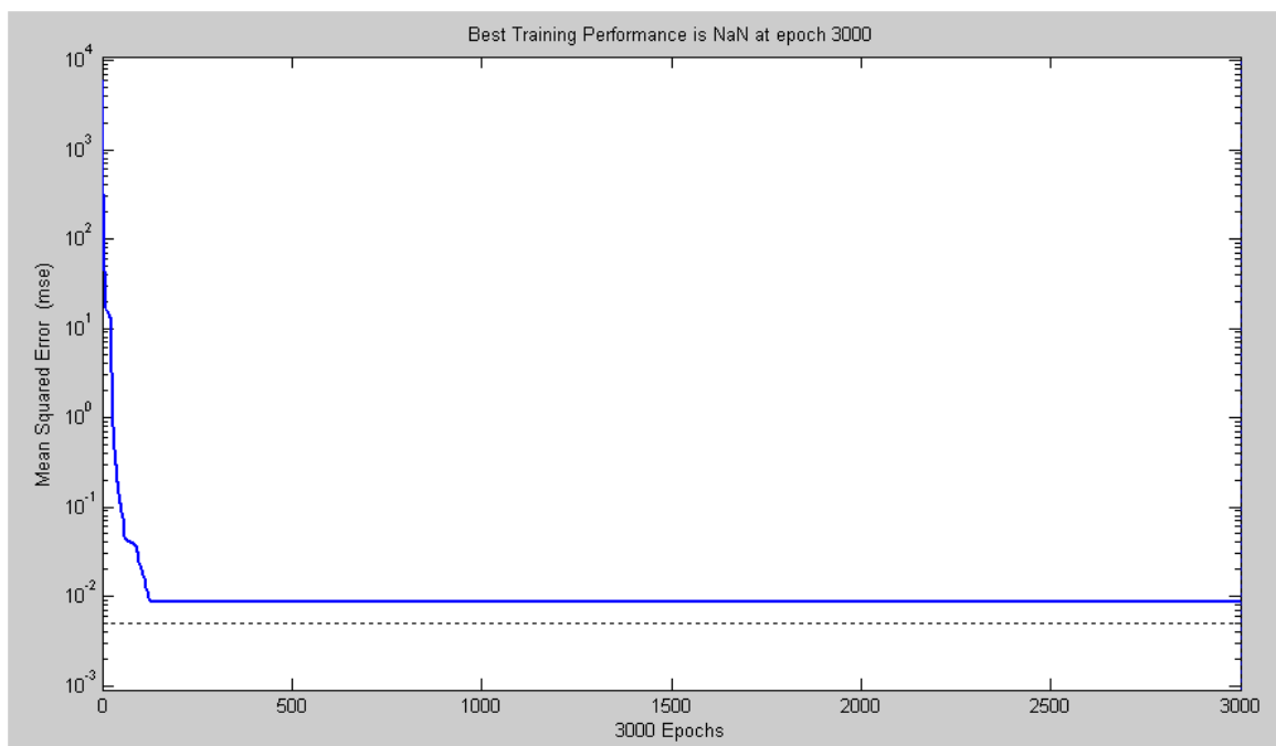
Figura 4.1 - Evolução do erro no processo de treinamento da RNA V.
