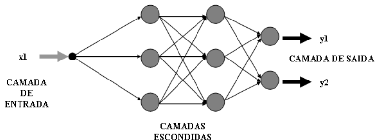
Figura 3.4 - Exemplo de rede feedforward (multicamadas).
